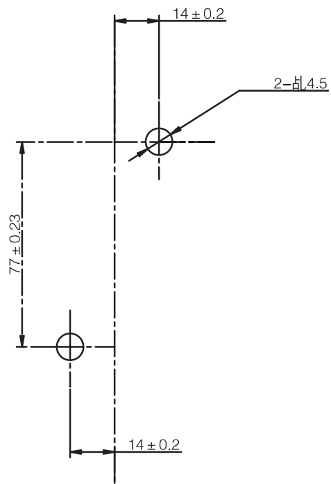
ABB系列（2S6C）板前接线开孔图
