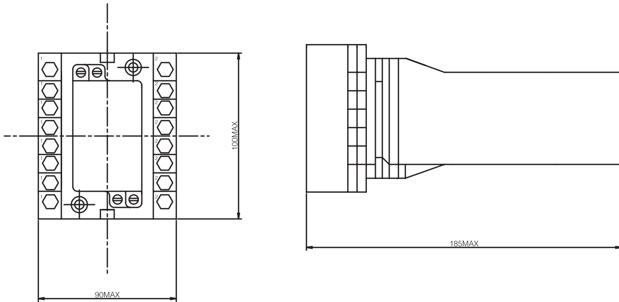
ABB系列（2S6C）板前接线外形图
