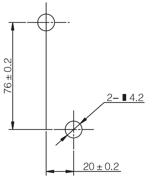
ABB系列（2S12C）板前接线外形图
