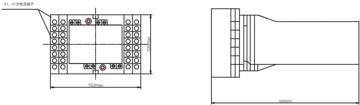
ABB系列（2S12C）板前接线外形图
