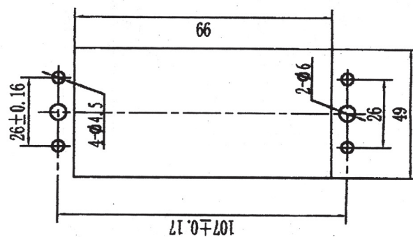
ABB-1U嵌入式开孔图
