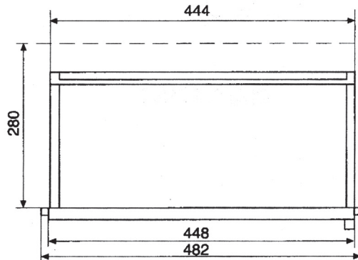
附图 9 安装继电器的设备框
