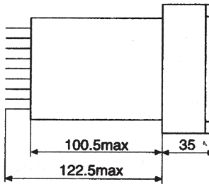
A11K (嵌入式板后接线)
