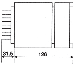
A11H (突出式板后接线)
