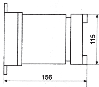
A11Q (突出式板前接线)
