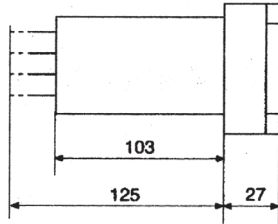
A01K (嵌入式板后接线)
