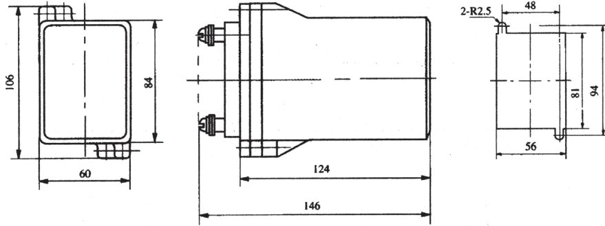
JK-1 壳体
